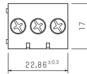
OTB-560-3P
