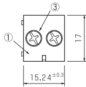
OTB-560-2P
